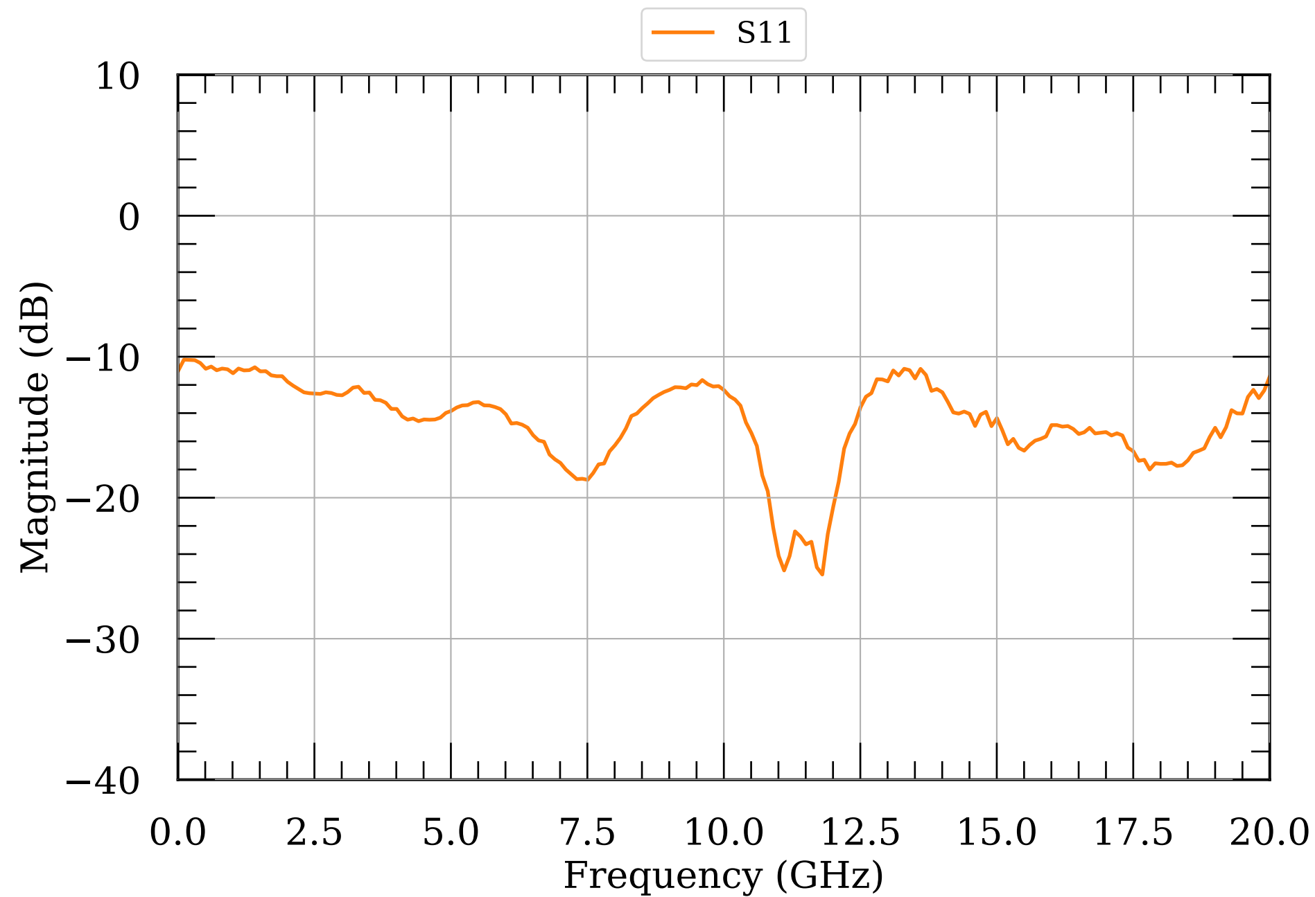
LNA S-params module025
